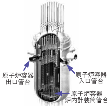
原子炉容器
